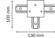
соединитель однофазный встраиваемый BARRA T-образный
