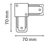
соединитель однофазный накладной BARRA L-образный
