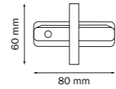
соединитель однофазный встраиваемый BARRA (малый) прямой
