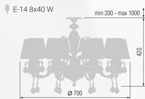
352 Chandelier 8-lamp Люстра 8-ми рожковая
