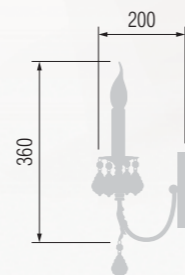
352 Wall lamp Бра однорожковое E-14 1x40 W
