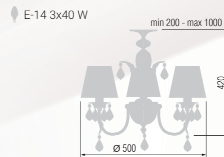
352 Chandelier 3-lamp Люстра 3-х рожковая
