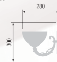
352 Wall lamp Бра однорожковое
