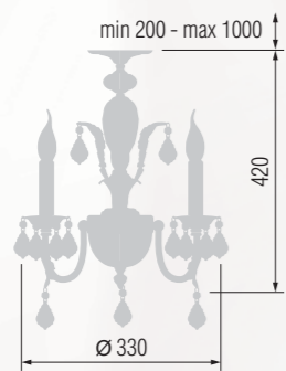
352 Chandelier 8-lamp Люстра 8-ми рожковая E-14 8x40 W
