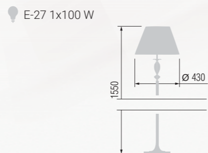
352 Floor lamp Торшер
